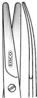
MAYO SCISSOR STR/COD T.C. TIP E-1463 - 6" STR E-1464 - 6" CUD E-1465 - 7" STR E-1466 - 7" CUD E-1467 - 8" STR E-1468 - 8" CUD
